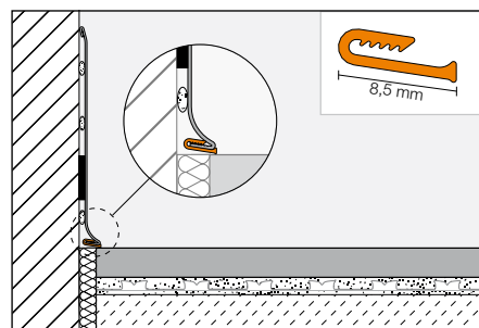
Lèvre d'étanchéité Schlüter®-DESIGNBASE-SLZ-E
